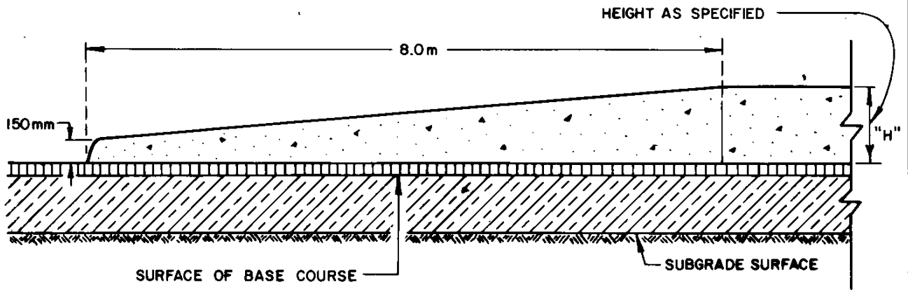
ELEVATION
