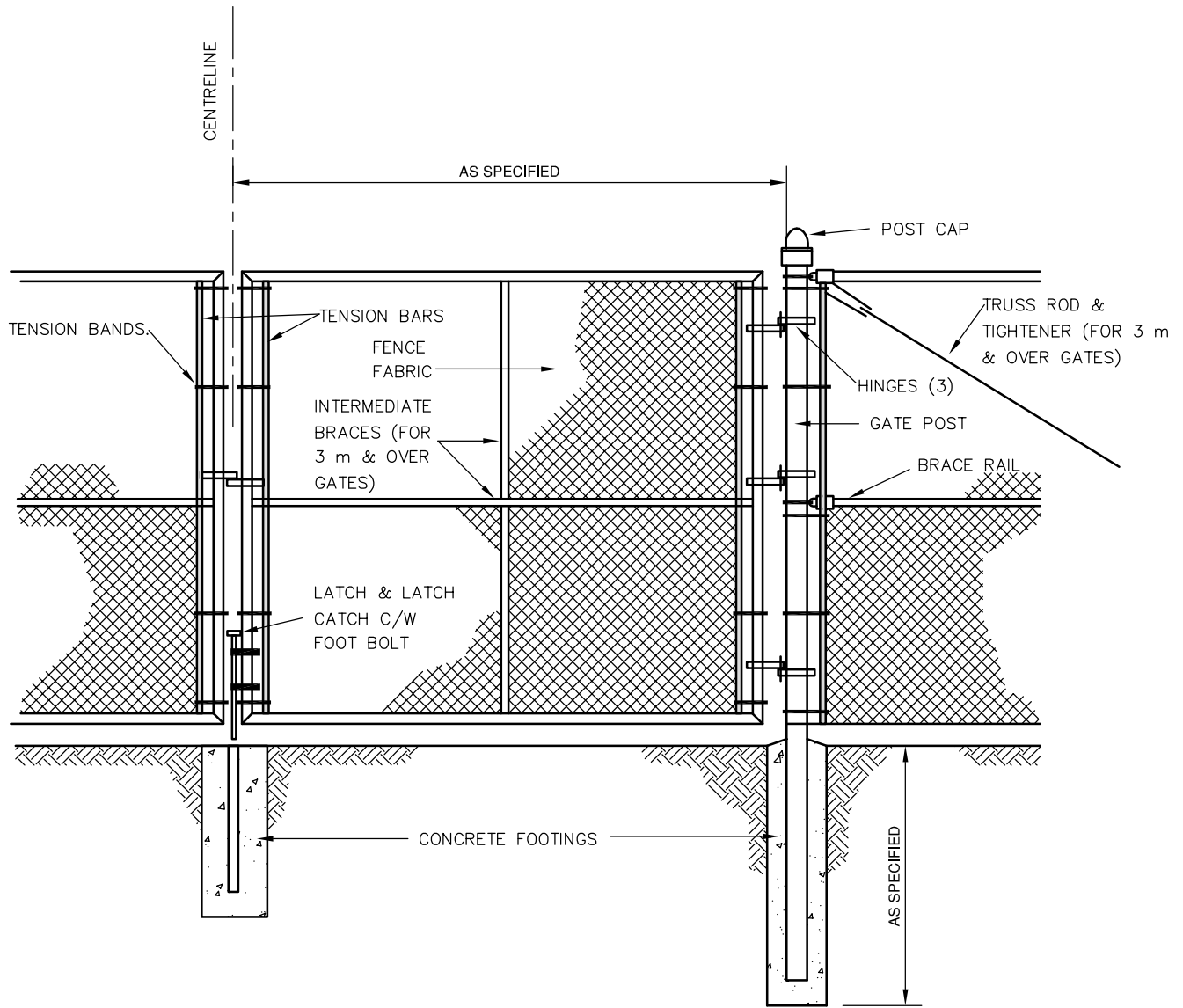
ELEVATION
