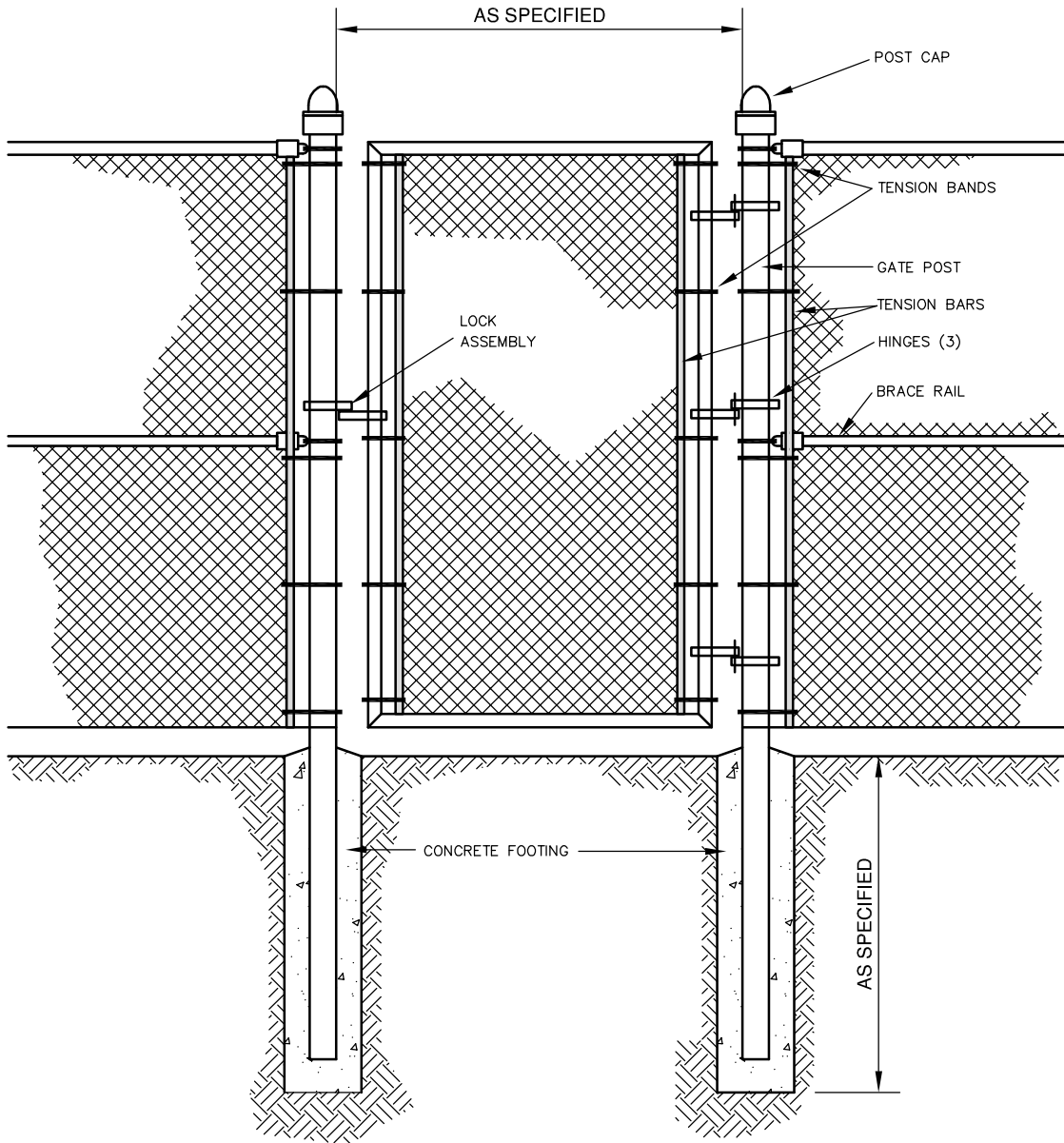
ELEVATION
