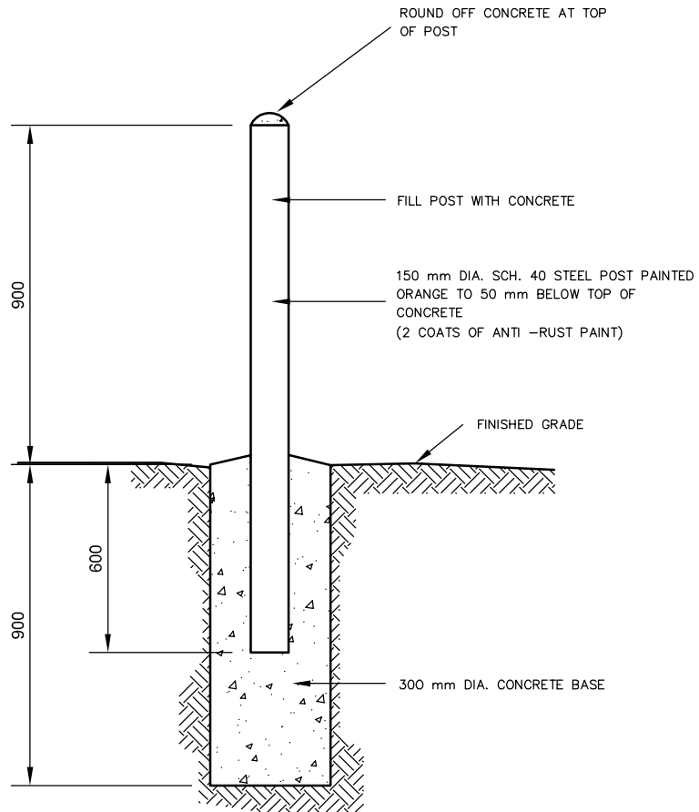
ELEVATION
