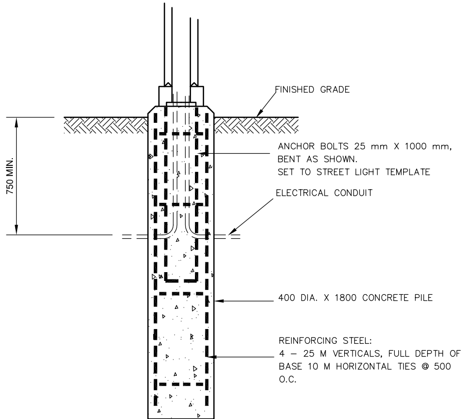
ELEVATION
